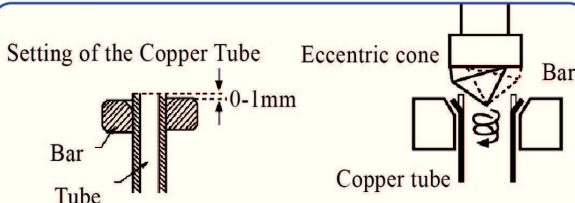
偏心扩管器 (45°) ECCENTRIC FLARING TOOL(45°)
